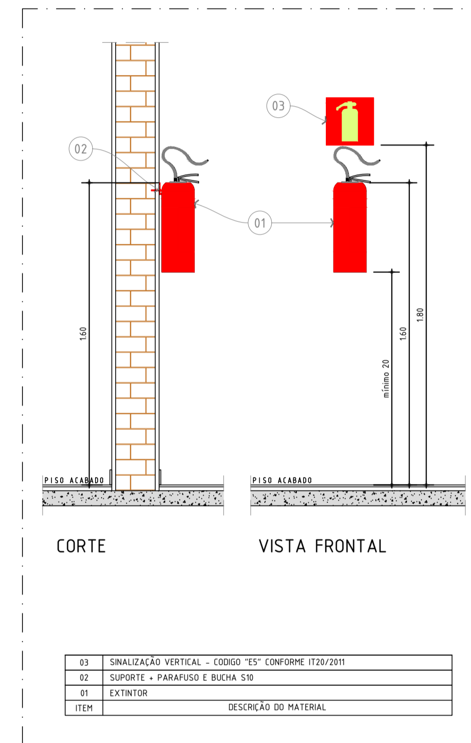
DET. TÍPICO EXTINTORES ESCALA 1:20
