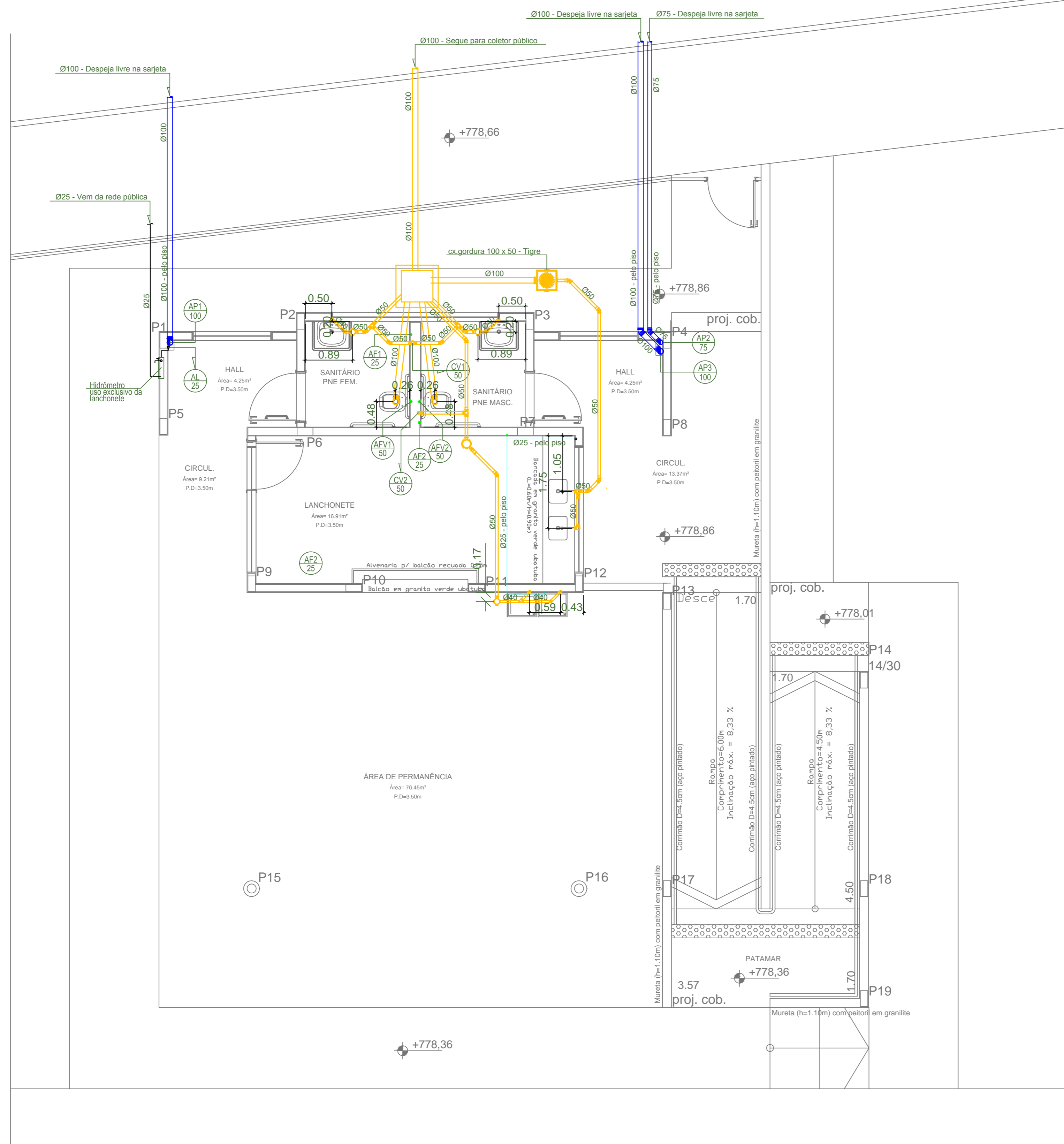
PLANTA DE DISTRIBUIÇÃO HIDRÁULICA - LANÇONETE - TÉRREO ESCALA: 1:50
