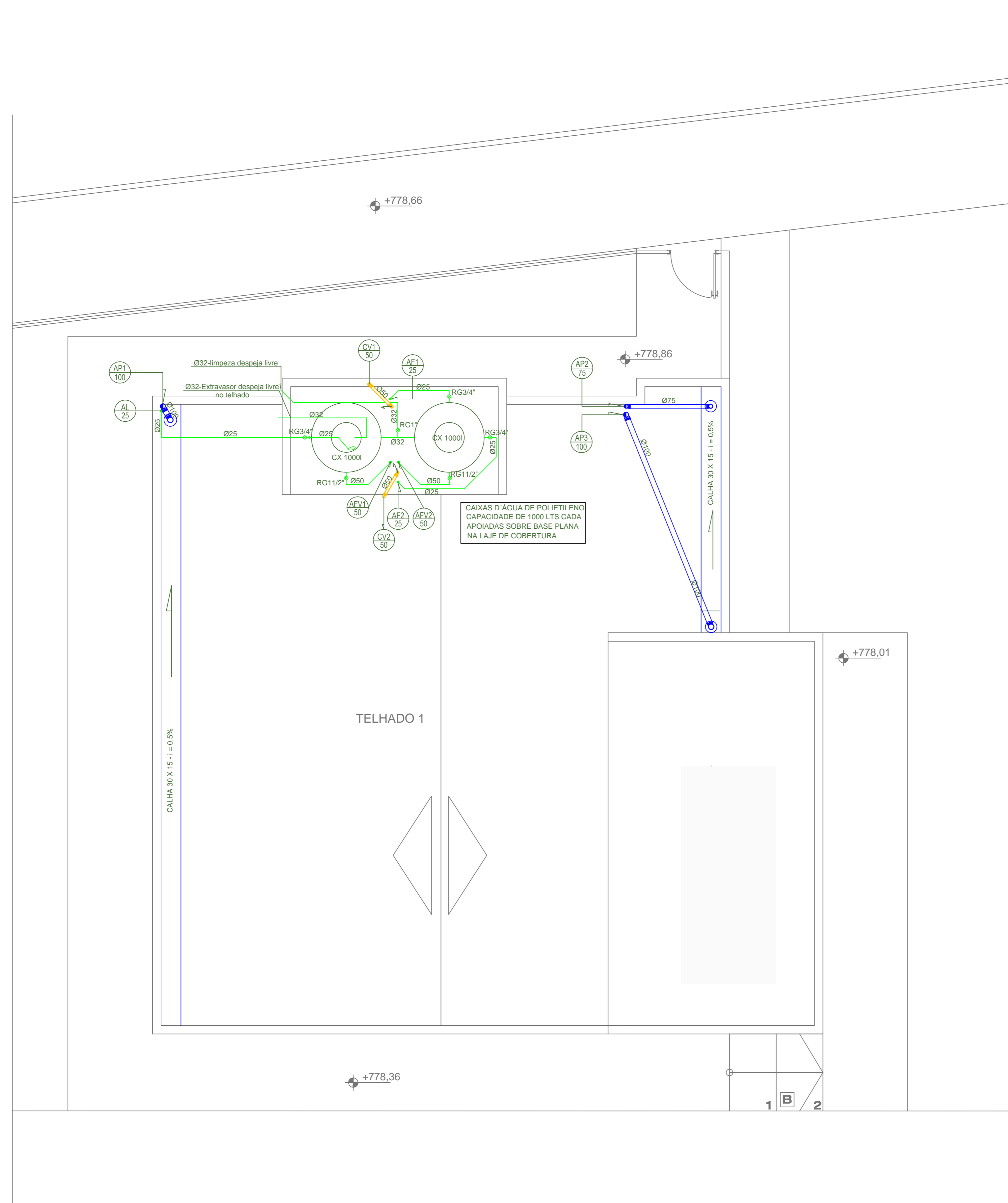
PLANTA DE DISTRIBUIÇÃO HIDRÁULICA - LANCHONETE - COBERTURA ESCALA: 1:50
