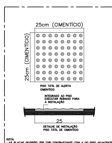
DETALHE PISO TÁTIL (SEM ESCALA)
