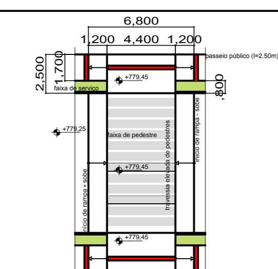
DETALHE TRAVESSIA ELEVADA DE PEDESTRES (SEM ESCALA)
