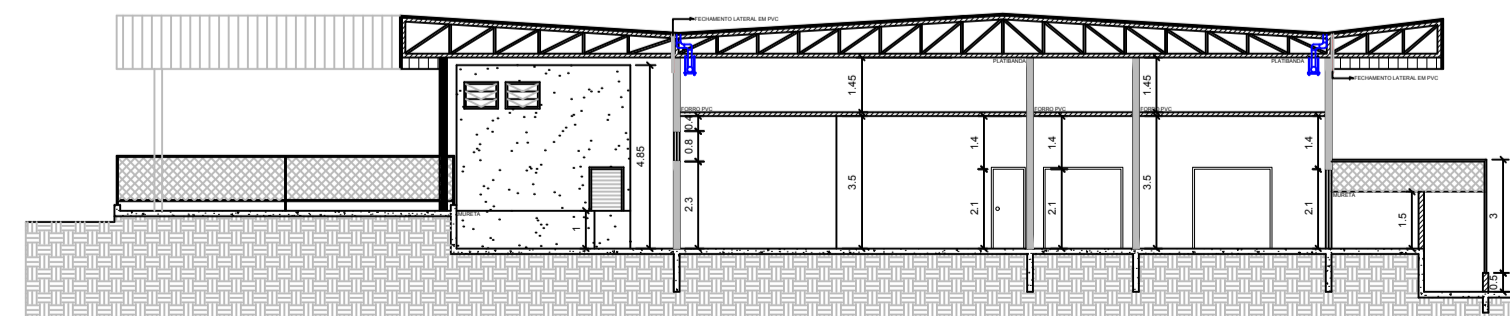
CORTE C C ESCALA 1/100
