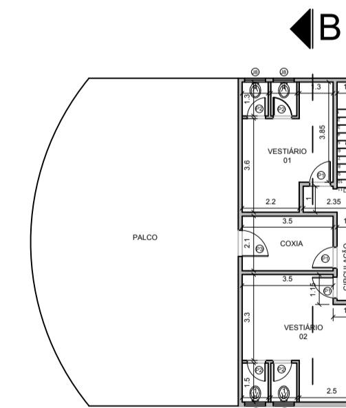
PLANTA BAIXA - SUPERIOR ESCALA 1/100
