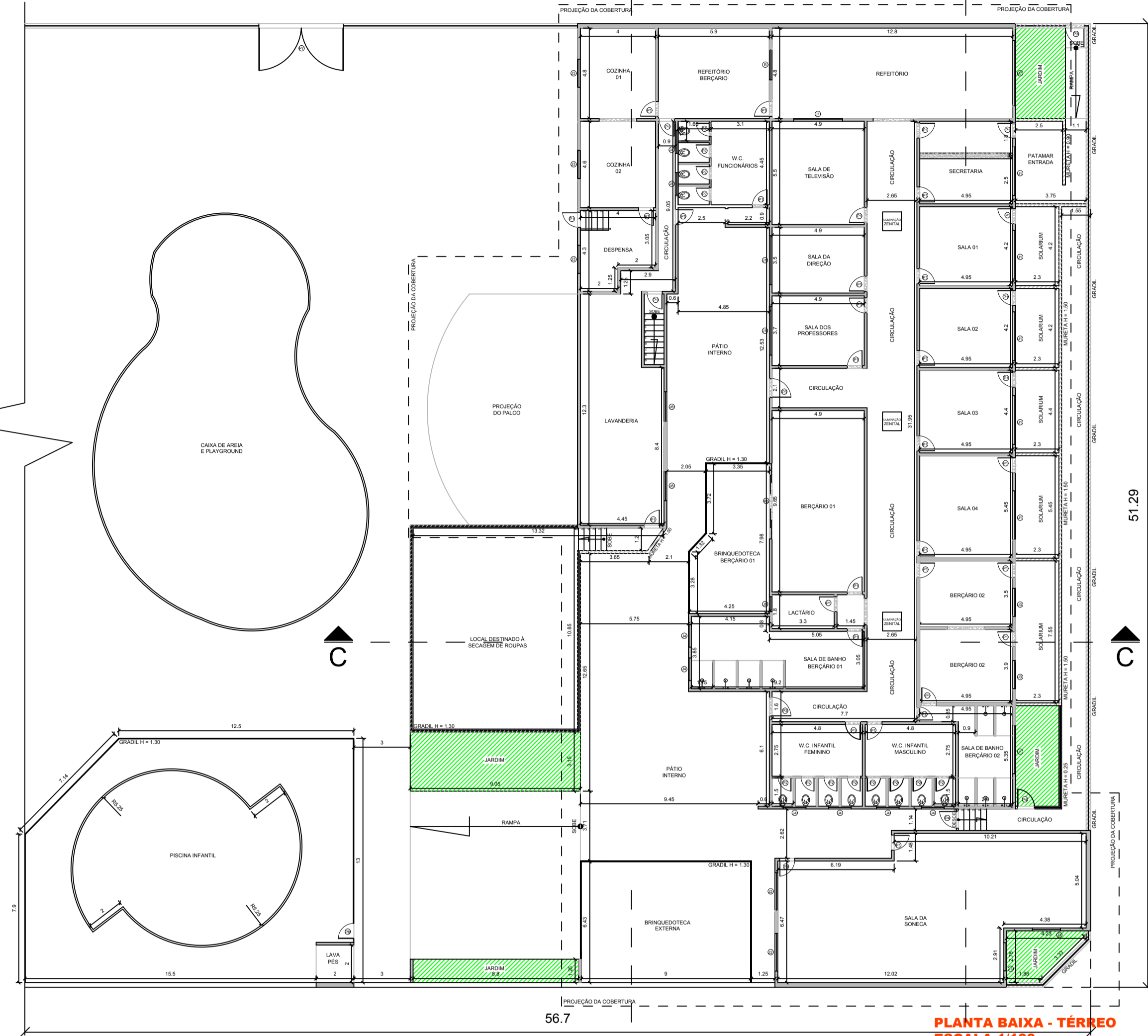
PLANTA BAIXA - TERRENO ESCALA 1/100
